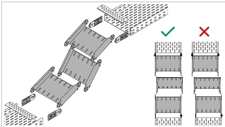
Obr. 69: Prvek kloubového oblouku s poloviční kloubovou spojkou a plechem dna
