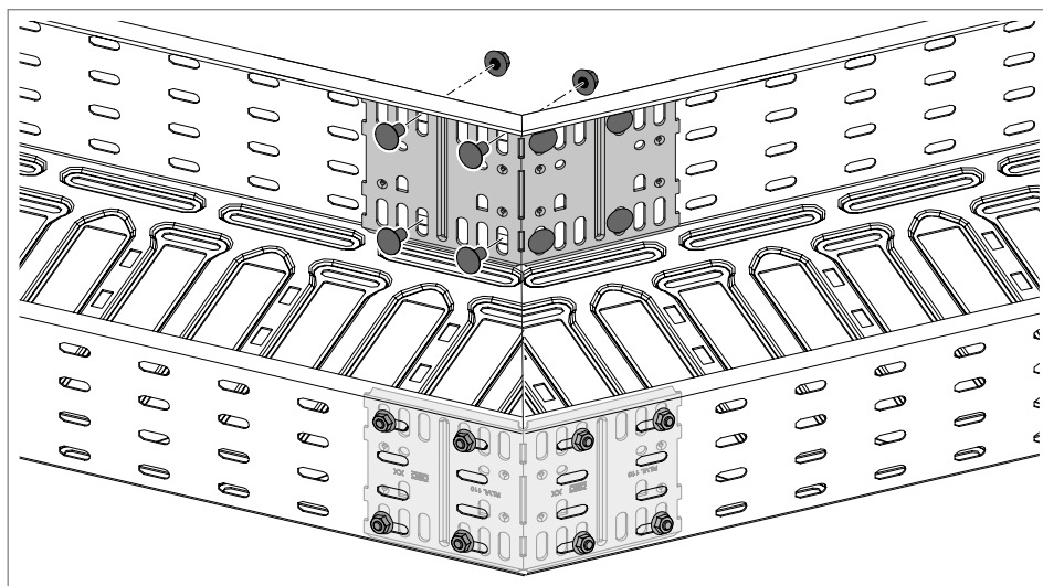
Obr. 32: Přišroubování podélné a úhlové spojky RLVL
