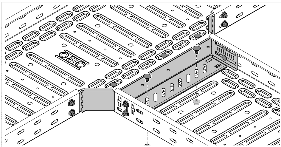
Obr. 57: Přišroubování odbočujícího kabelového žlabu k vestavnému odbočnému dílu
