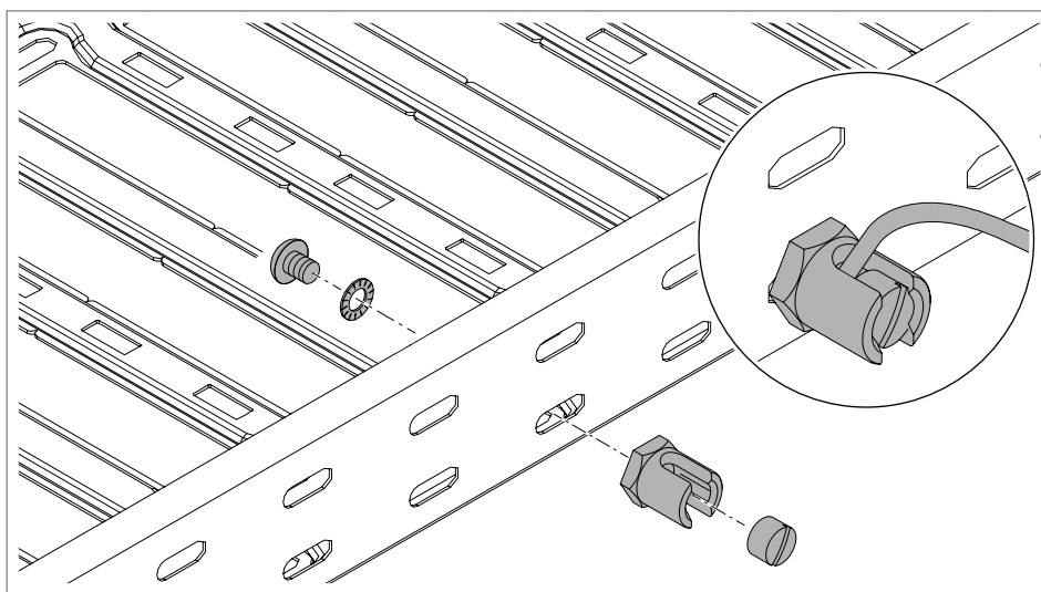
Obr. 82: Montáž uzemňovací svorky
