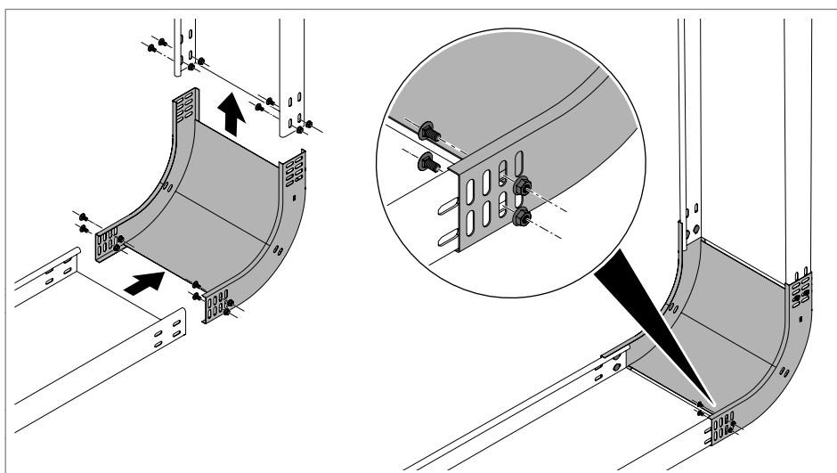
Obr. 68: Montáž stoupajícího svislého oblouku
