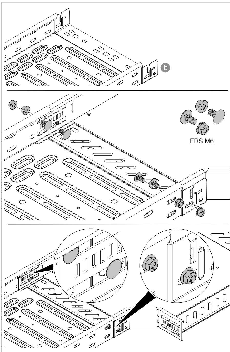
Obr. 49: Upevnění tvarového dílu pomocí šroubů (nedělenému žlabu (b))
