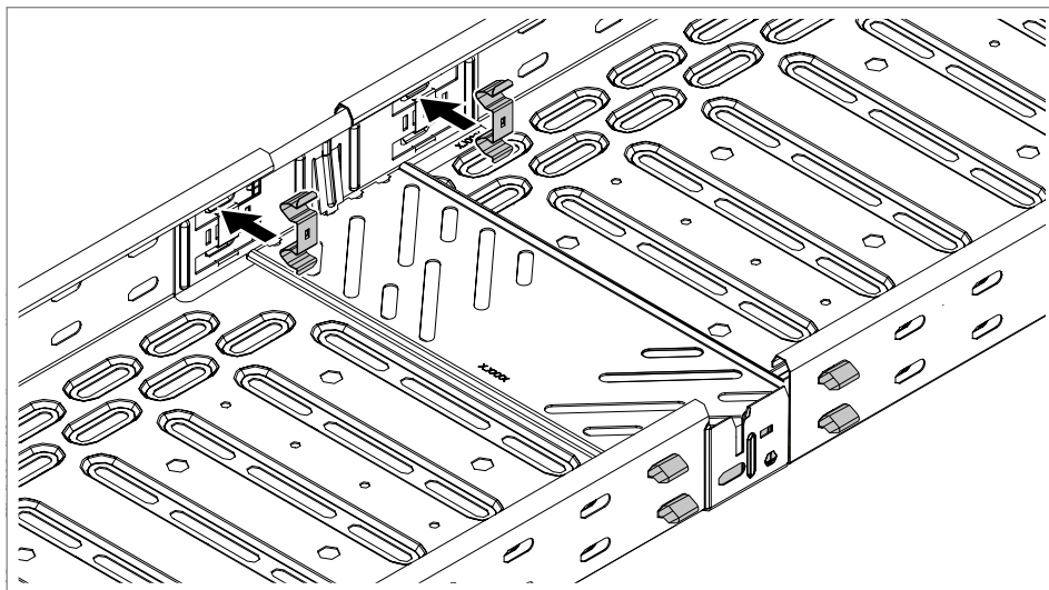
Obr. 24: Upevnění spojky dvojitými svorkami
