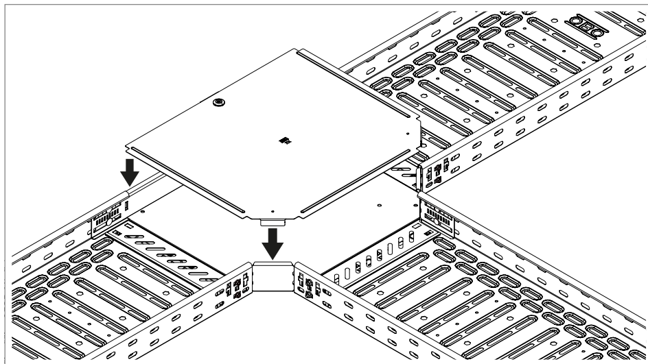
Obr. 90: Nasazení víka tvarového dílu
