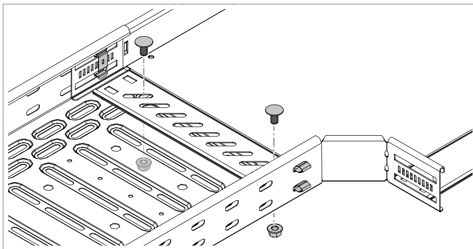
Obr. 52: Přišroubování spojuvací lišty
