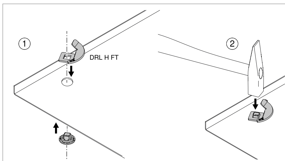
Obr. 88: Přinýtování otočné západky
