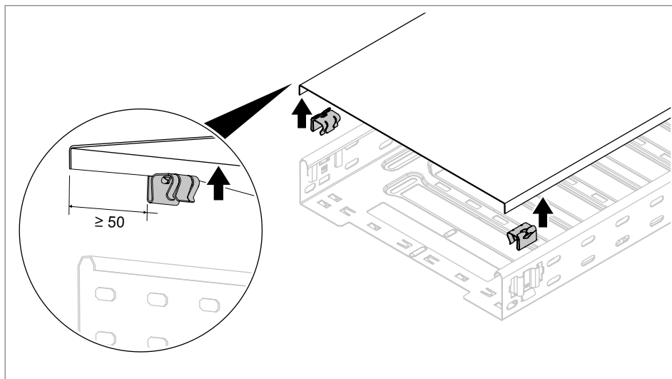
Obr. 83: Upnutí spony víka k víku
