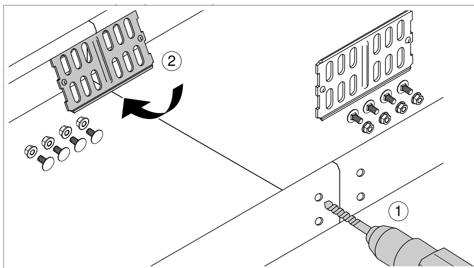
Obr. 25: Nasazení podélné spojky RLVK
