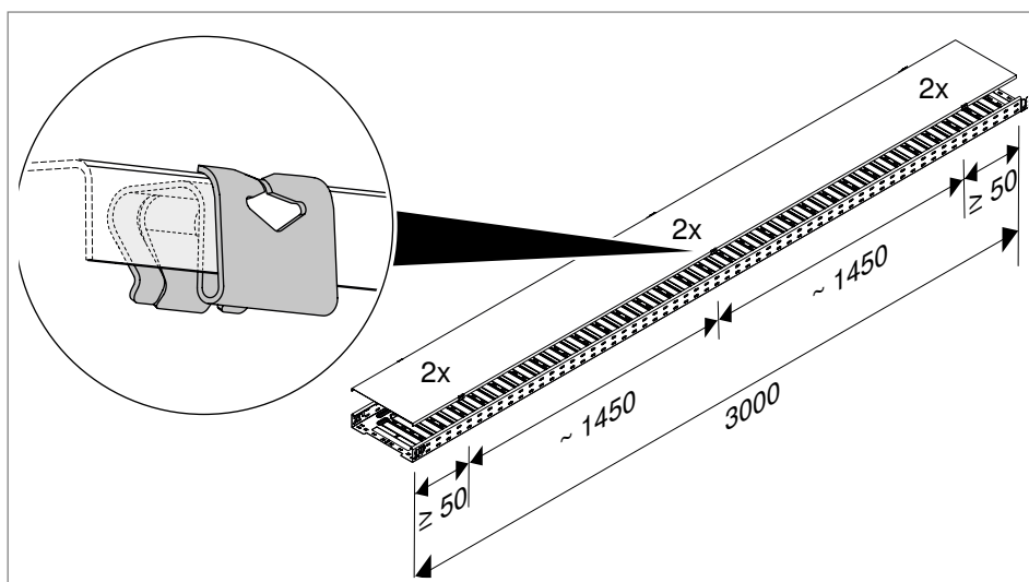
Obr. 84: Rozložení potřebného počtu spon víka
