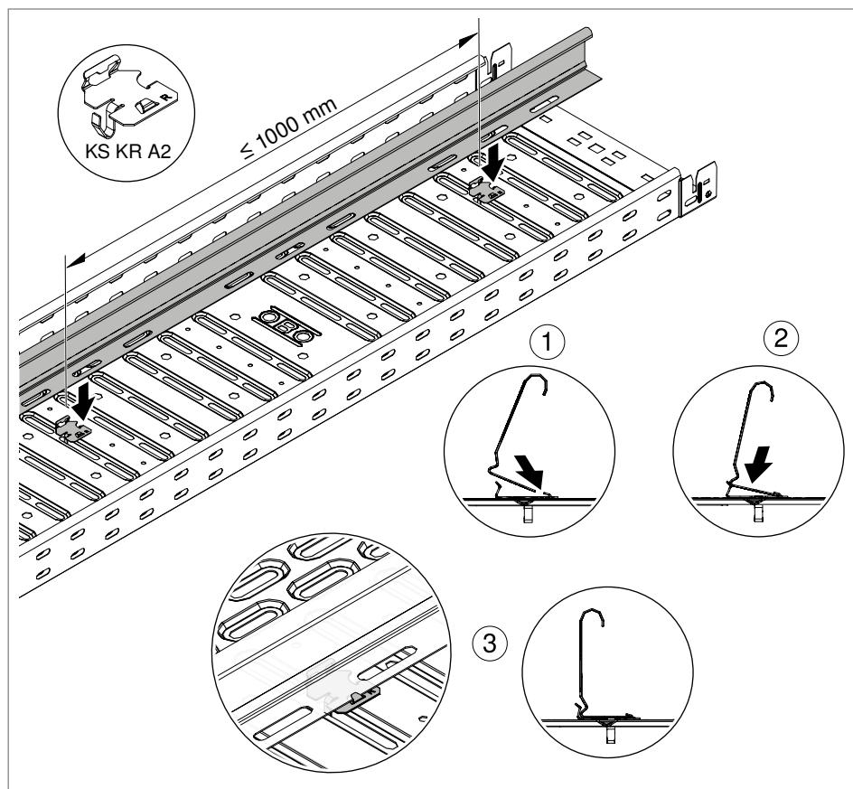
Obr. 80: Nasazení přepážky do svorky
