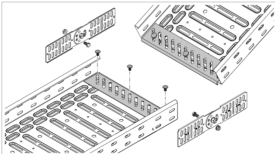
Obr. 39: Přišroubování plechů dna
