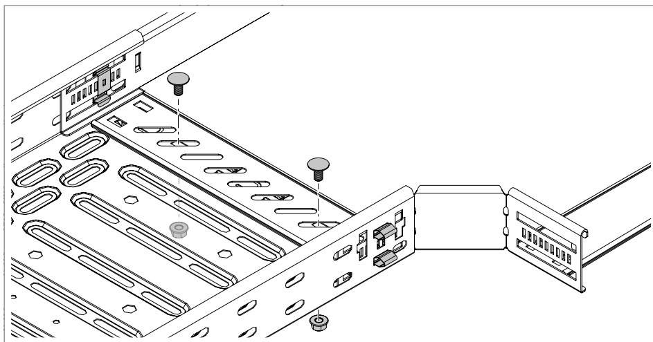
Obr. 47: Přišroubování spojuvací lišty
