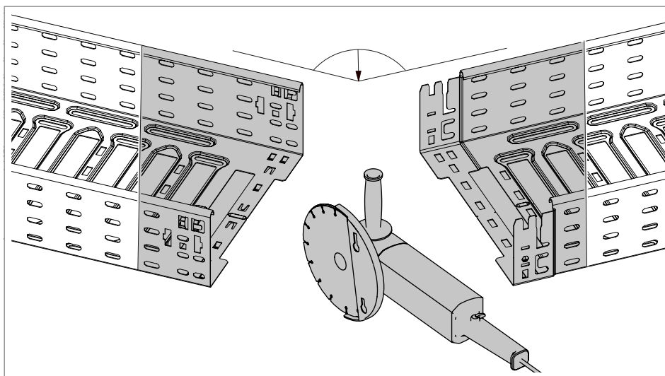
Obr. 30: Zařízení kabelového žlabu pro zhotovení úhlu
