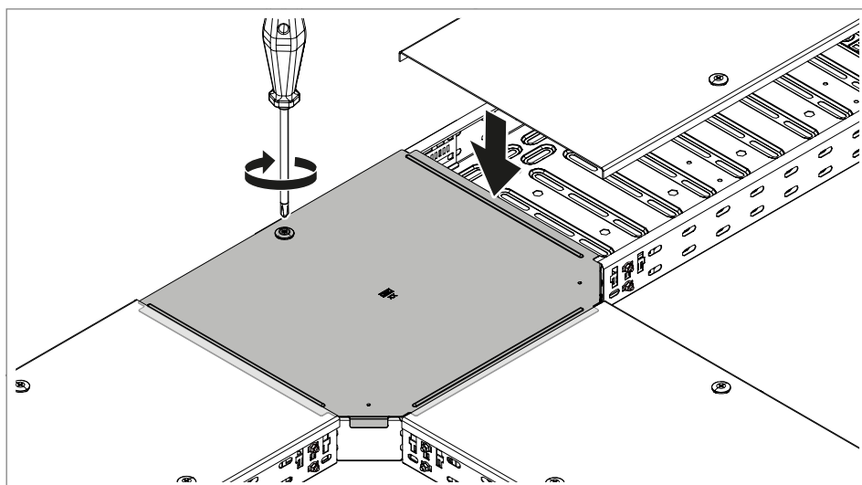
Obr. 91: Zajištění víka tvarového dílu víkem trasy
