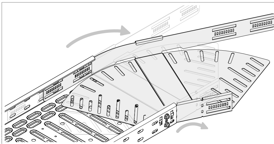
Obr. 62: Ohnutí oblouku s nastavitelným úhlem
