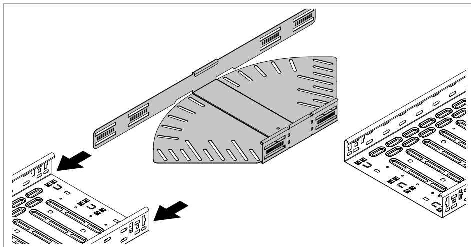
Obr. 60: Zasunutí oblouku s nastavitelným úhlem
