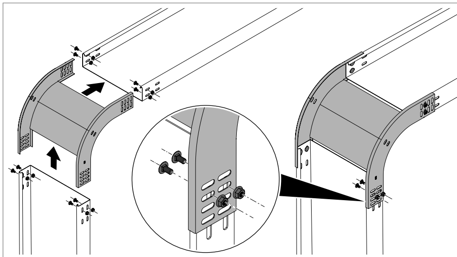
Obr. 67: Montáž klesajícího svislého oblouku
