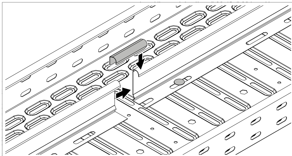
Obr. 81: Spojení přepážek
