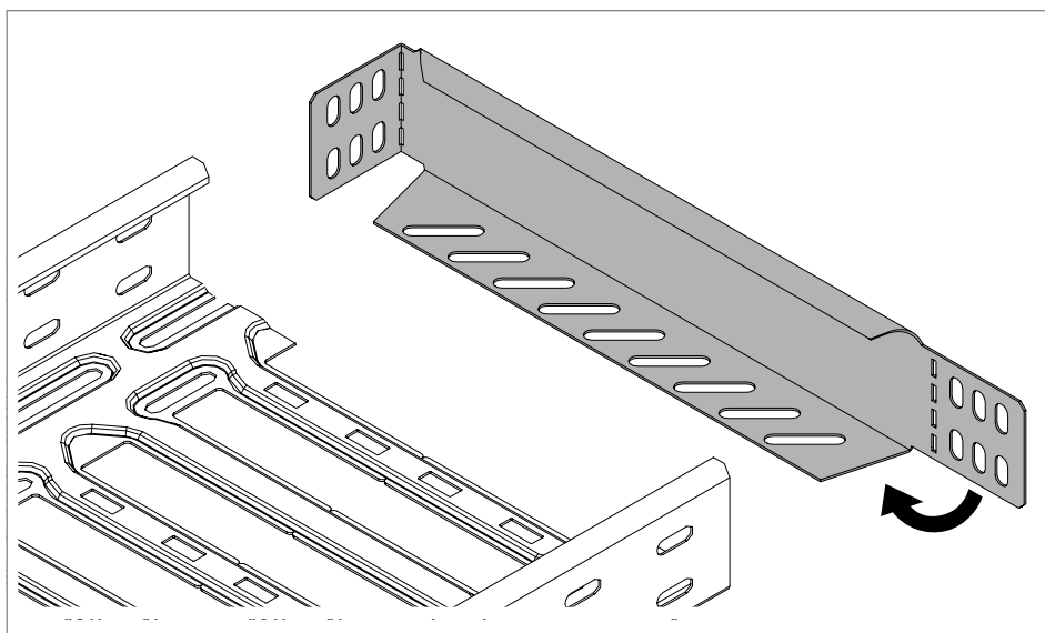
Obr. 76: Ohnutí jazýčku
