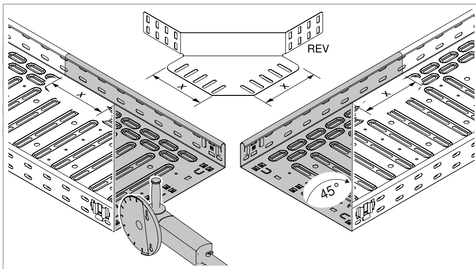
Obr. 36: Zařízení kabelových žlabů pro rohovou spojku REV
