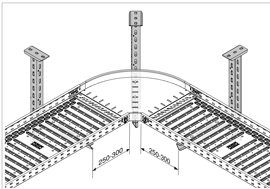
Obr. 44: Příklad podepření tvarového dílu: 90° oblouk šířky 400 mm
