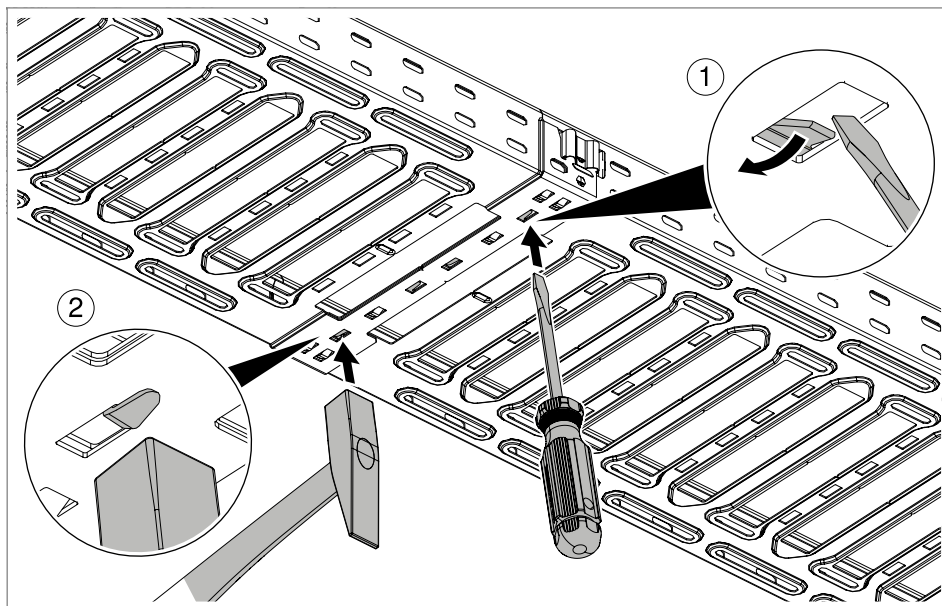
Obr. 20: Zajištění spojení žlabů
