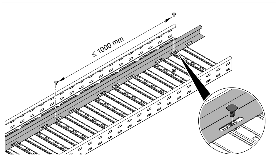
Obr. 78: Přišroubování přepážky
