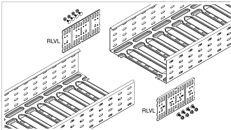
Obr. 27: Podélná spojka RLVL
