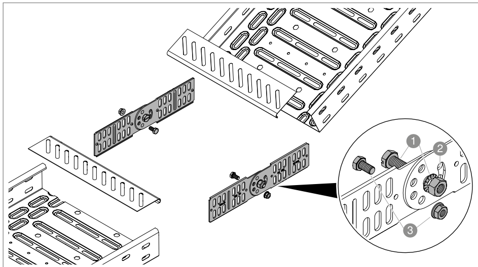
Obr. 38: Kloubová spojka RGV a plechy dna
