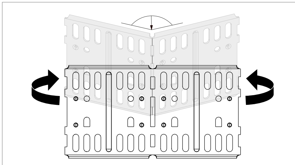
Obr. 31: Ohnutí podélné a úhlové spojky RLVL
