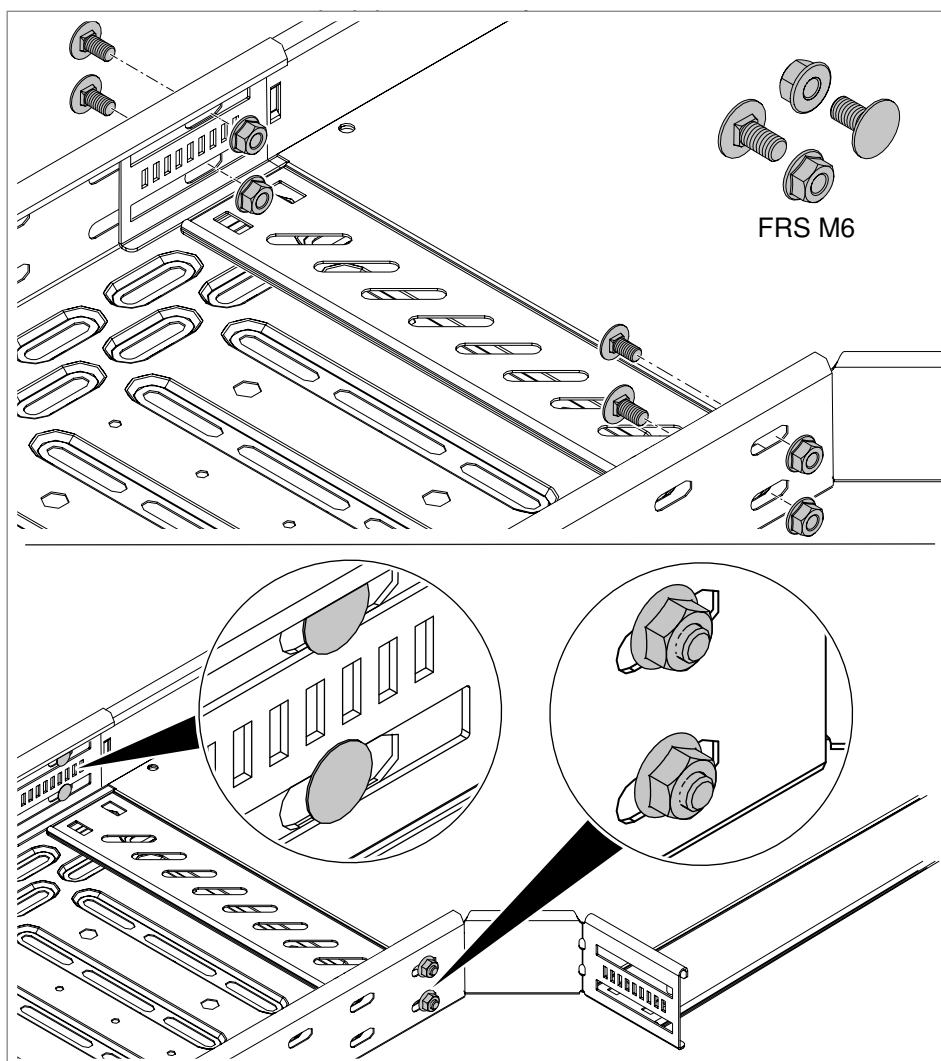
Obr. 53: Upevnění tvarového dílu pomocí dvojité svorky
