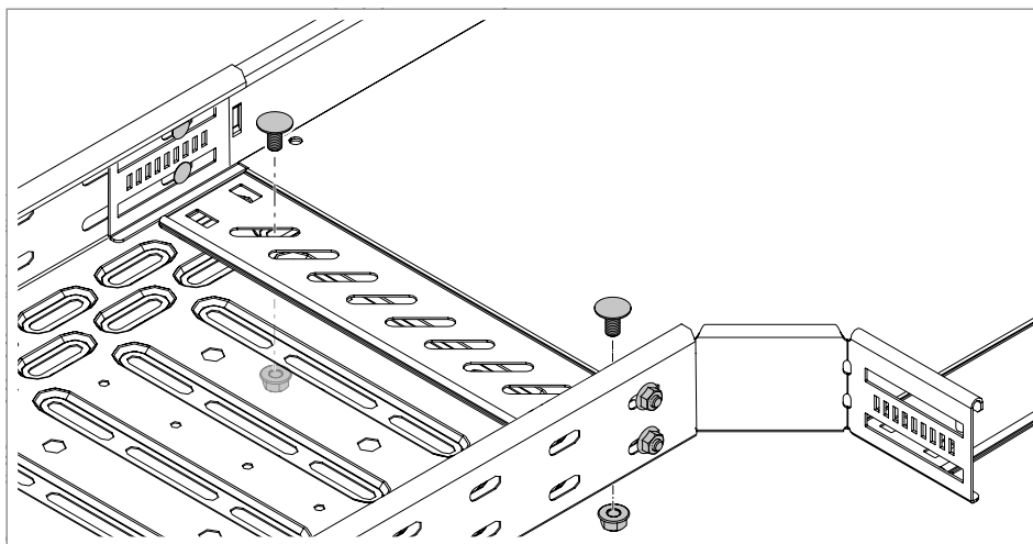
Obr. 54: Přišroubování spořovací lišty
