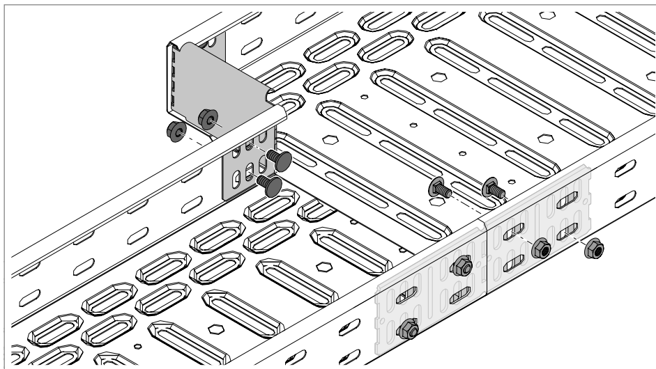
Obr. 74: Montáž podélné a úhlové spojky a redukčního úhelníku
