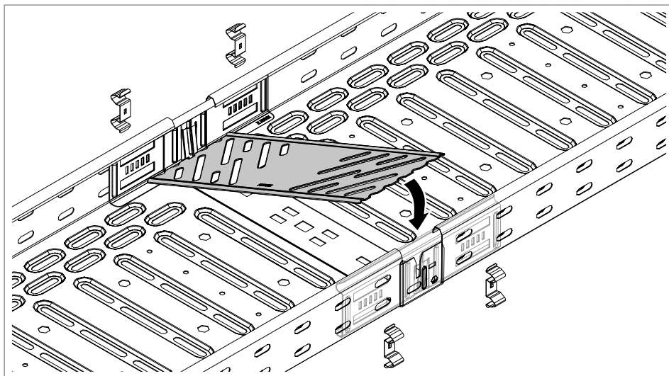
Obr. 23: Nasazení spojovací lišty podélné spojky KTSM
