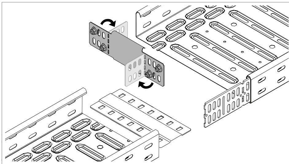
Obr. 73: Ohnutí redukčního úhelníku
