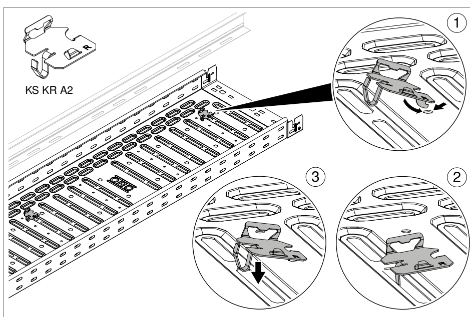
Obr. 79: Nasazení svorky pro přepážku
