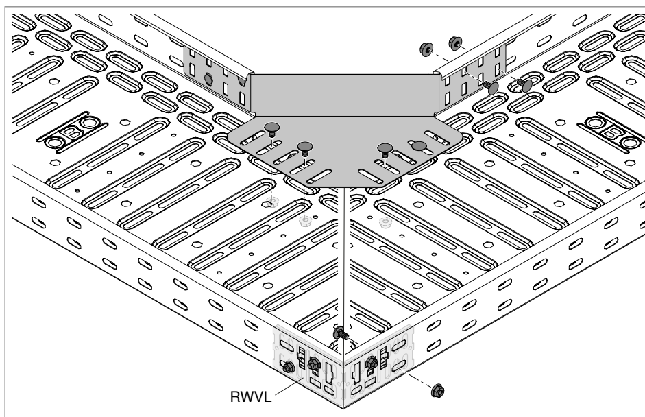
Obr. 37: Montáž rohové spojky REV
