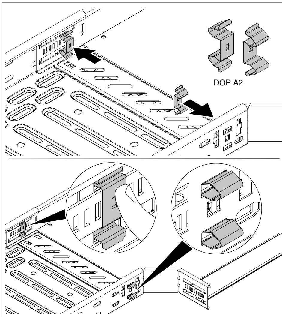
Obr. 46: Upevnění tvarového dílu pomocí dvojité svorky
