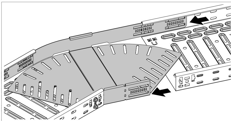
Obr. 63: Nasunutí druhého žlabu na oblouk
