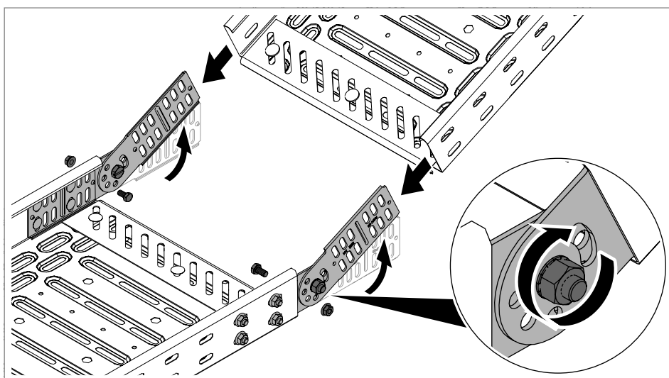
Obr. 41: Dotažení kloubového šroubu
