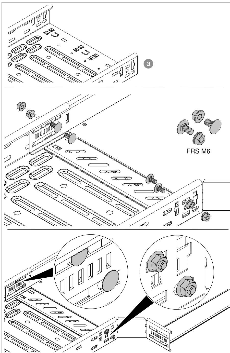
Obr. 48: Upevnění tvarového dílu pomocí šroubů (nedělenému žlabu (a))
