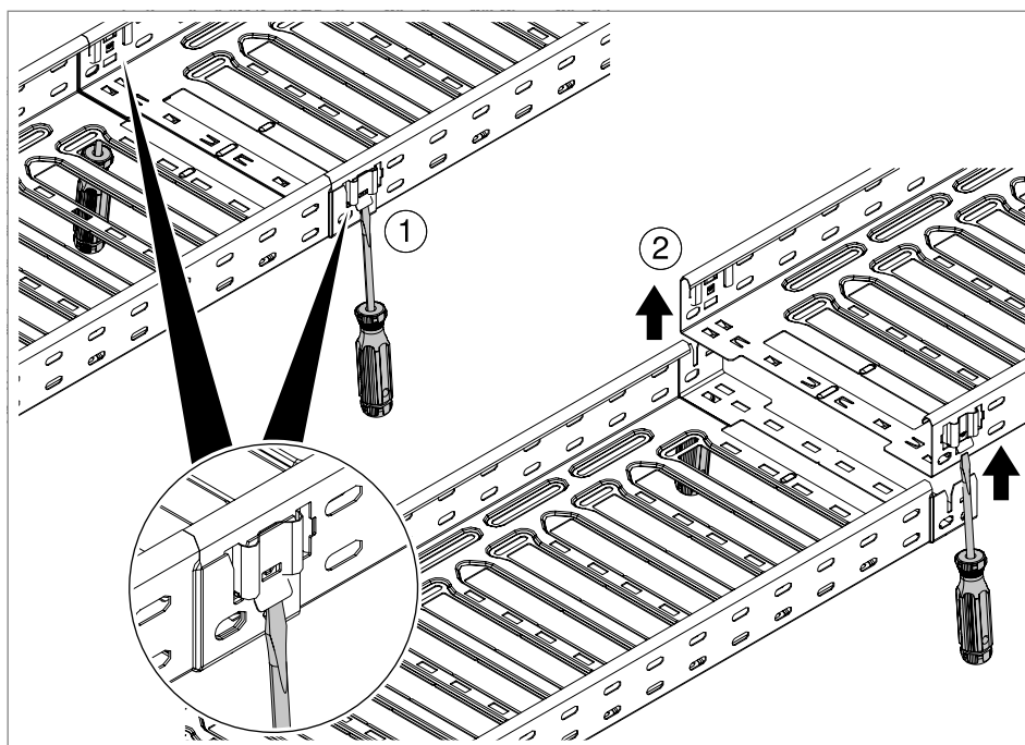
Obr. 92: Opětovné uvolnění násuvného spojení Magic
