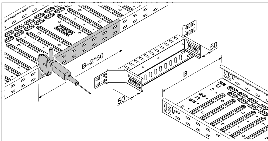
Obr. 55: Vylomení bočnice kabelového žlabu
