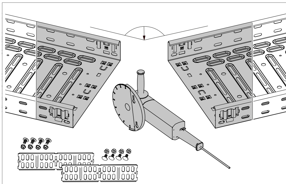
Obr. 33: Zařízení kabelového žlabu pro zhotovení úhlu
