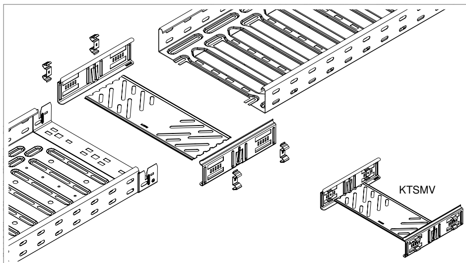
Obr. 21: Podélná spojka KTSM
