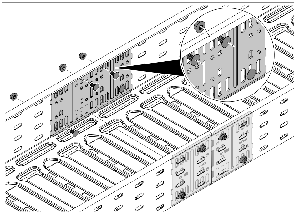
Obr. 29: Přišroubování podélné spojky RLVL
