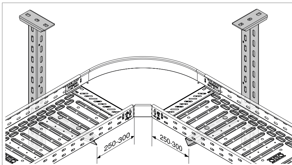
Obr. 43: Příklad podepření tvarového dílu: 90° oblouk šířky 300 mm
