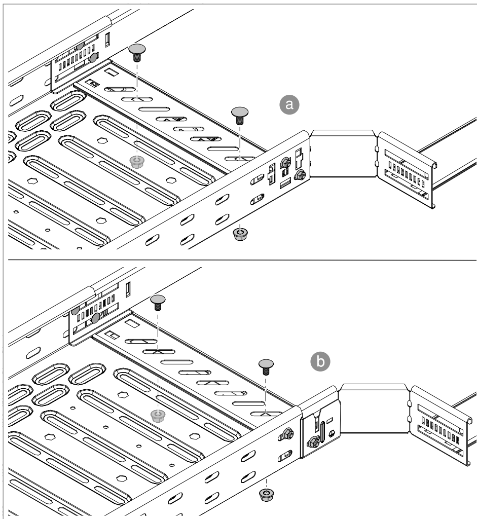
Obr. 50: Přišroubování spojovací lišty (nedělenému žlabu a a b )
