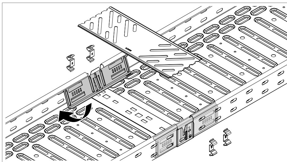
Obr. 22: Nasazení podélné spojky KTSM
