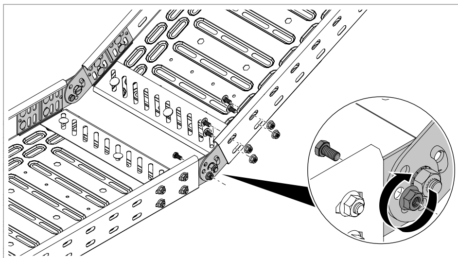
Obr. 42: Dotažení pojistného šroubu
