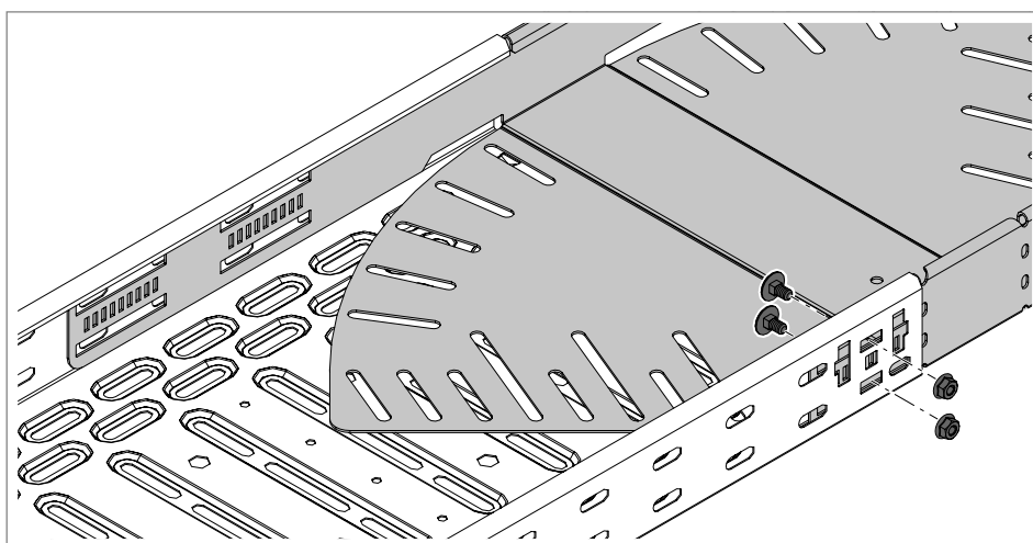
Obr. 61: Upevnění oblouku s nastavitelným úhlem
