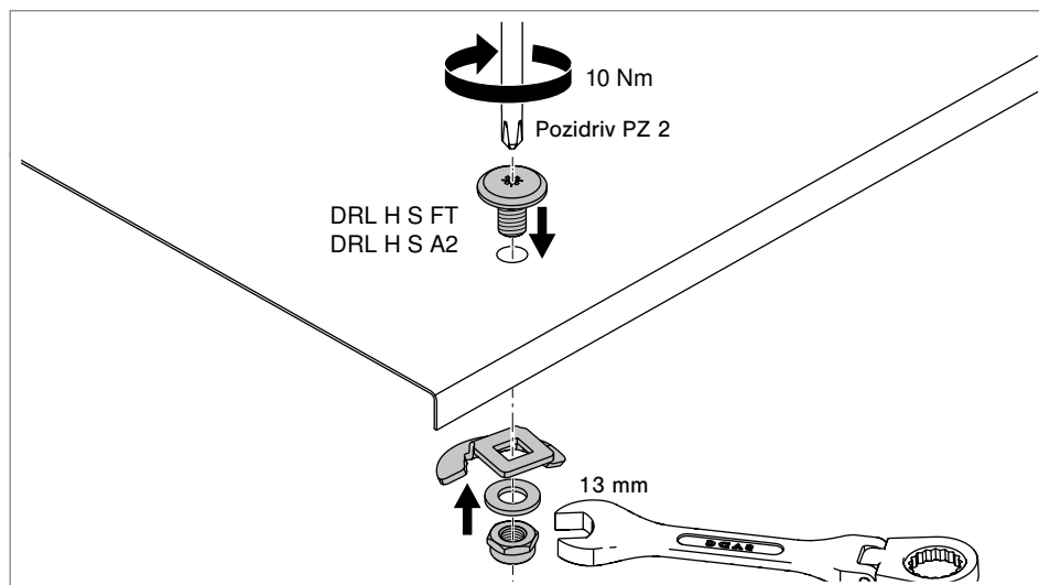
Obr. 87: Přišroubování otočné západky
