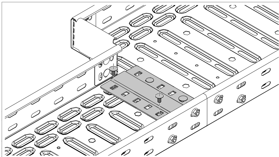
Obr. 75: Přišroubování spojovací lišty
