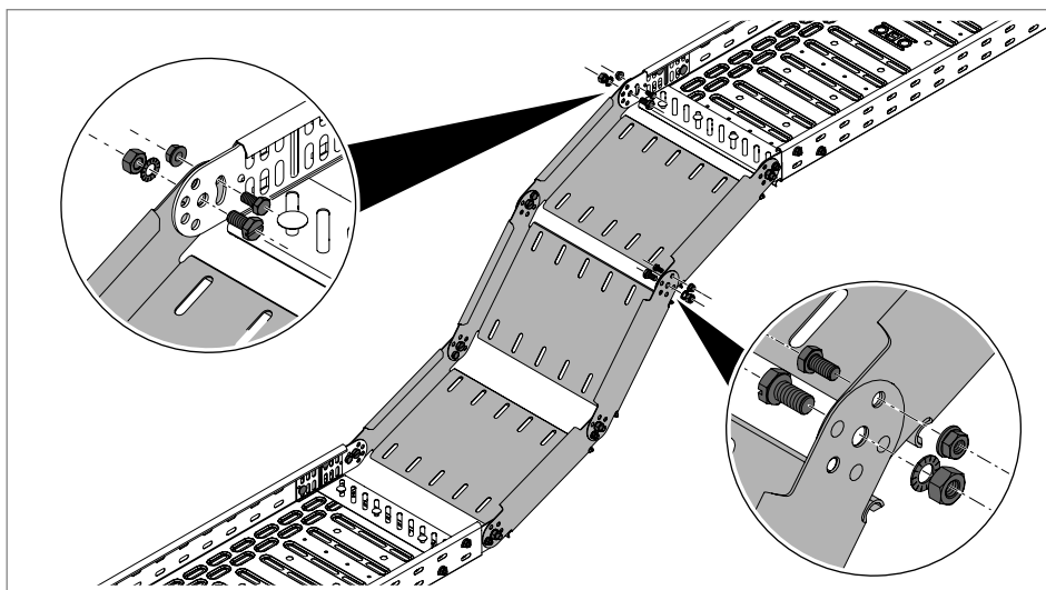
Obr. 72: Montáž prvků kloubového oblouku
