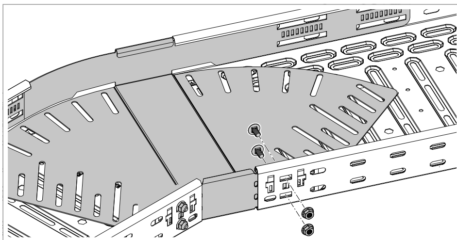
Obr. 64: Upevnění druhého žlabu k oblouku
