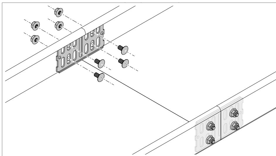
Obr. 26: Přišroubování podélné spojky RLVK
