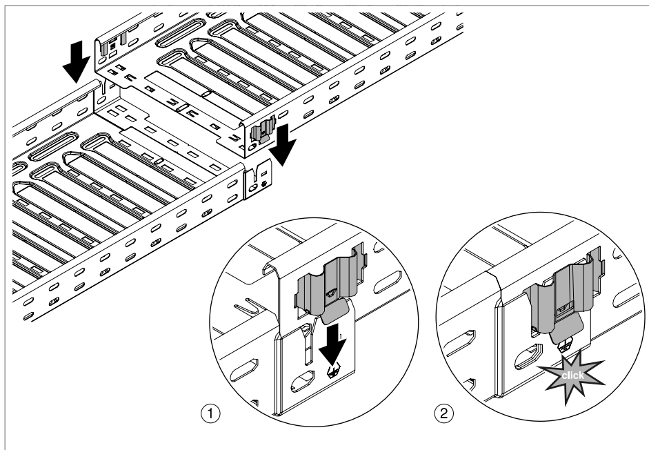
Obr. 19: Násuvná spojka Magic s pružinovým prvkem
