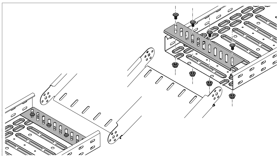
Obr. 70: Montáž plechu dna
