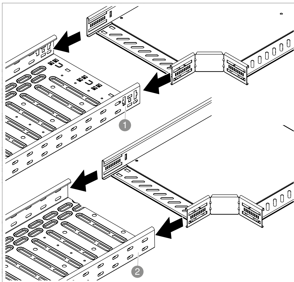
Obr. 45: Zasunutí tvarového dílu
