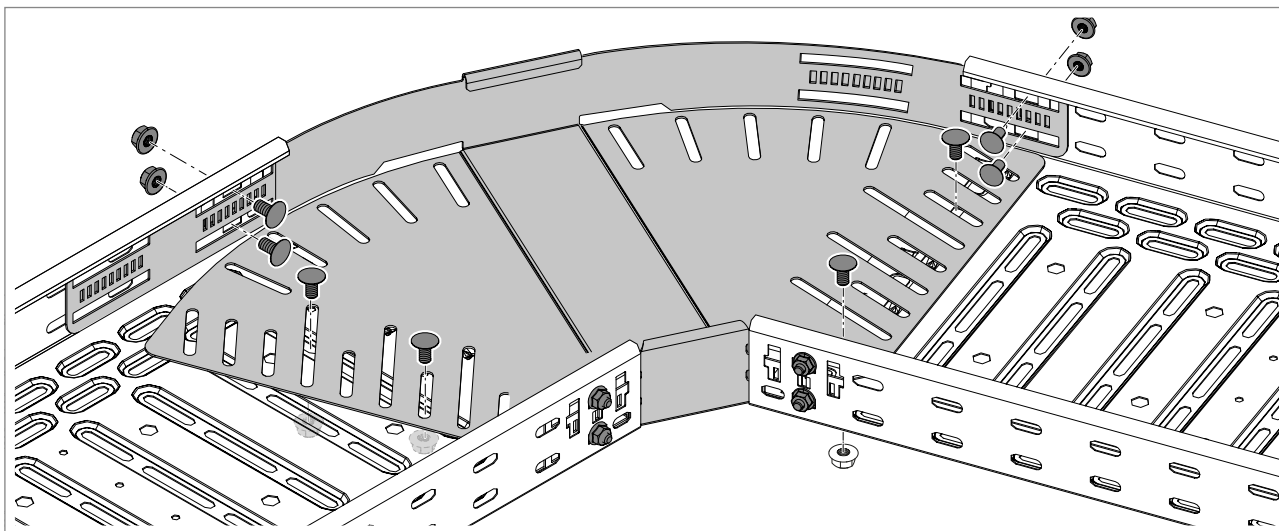
Abb. 66: Přišroubování spojek a míst styku ke žlabům
