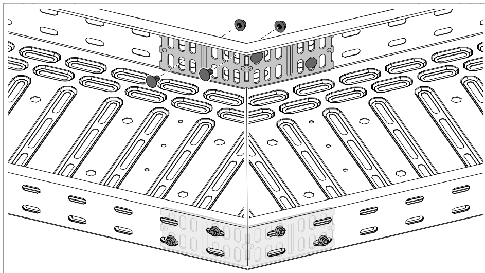
Obr. 35: Přišroubování úhlové spojky RWVL
