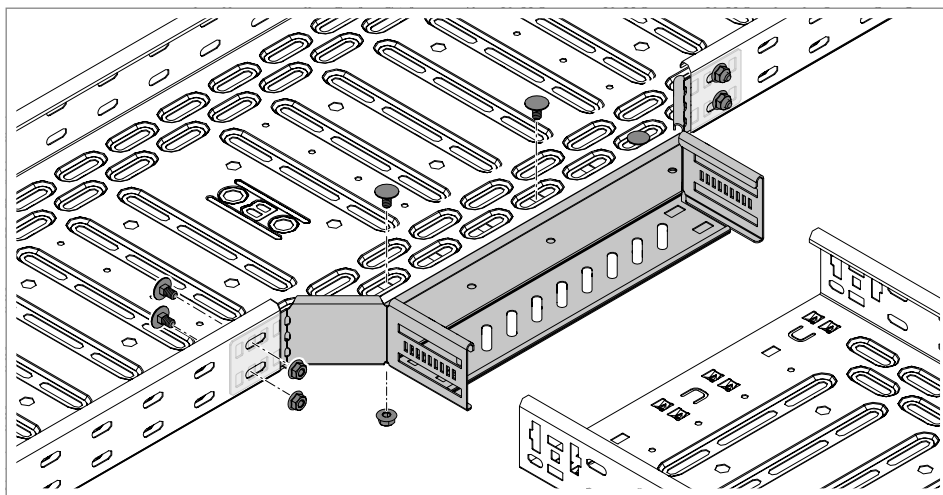
Obr. 56: Přišroubování vestavného odbočného dílu k nedělenému kabelovému žlabu
