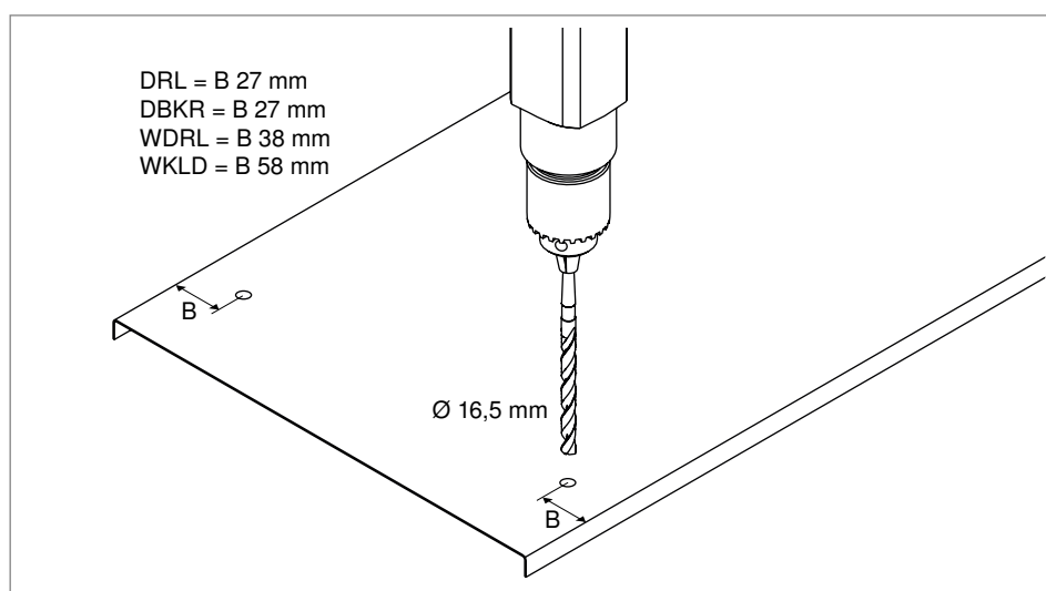
Obr. 86: Předvrtání otvorů do víka
