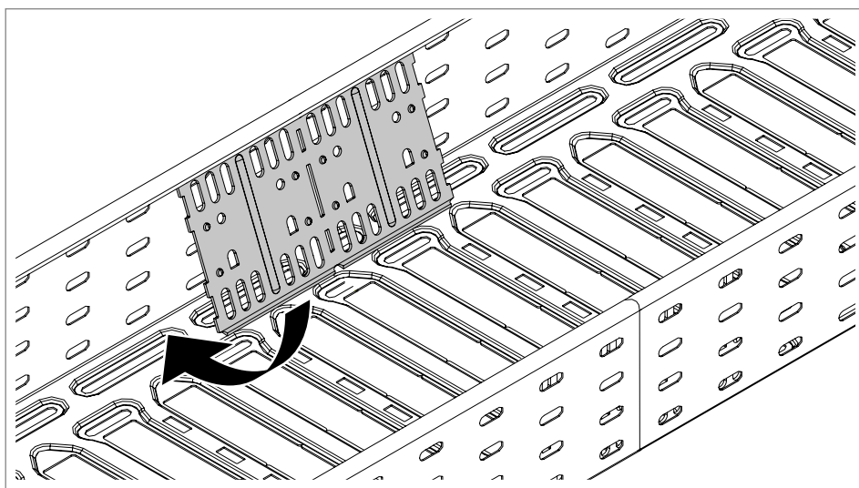
Obr. 28: Nasazení podélné spojky RLVL
