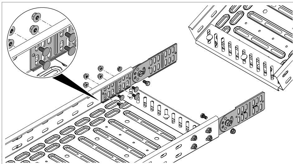
Obr. 40: Přišroubování kloubové spojky RGV ke kabelovému žlabu
