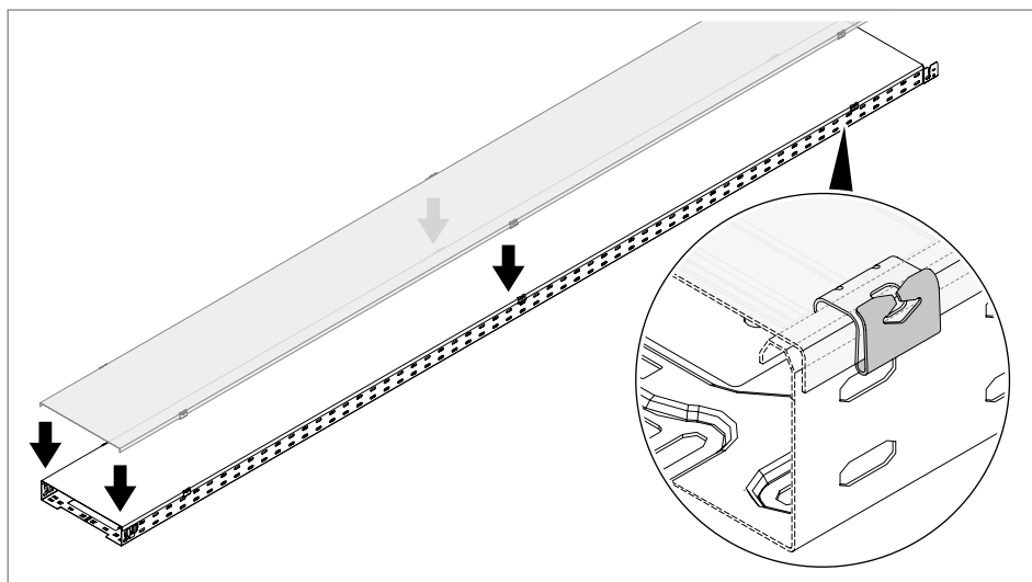
Obr. 85: Naklapnutí víka
